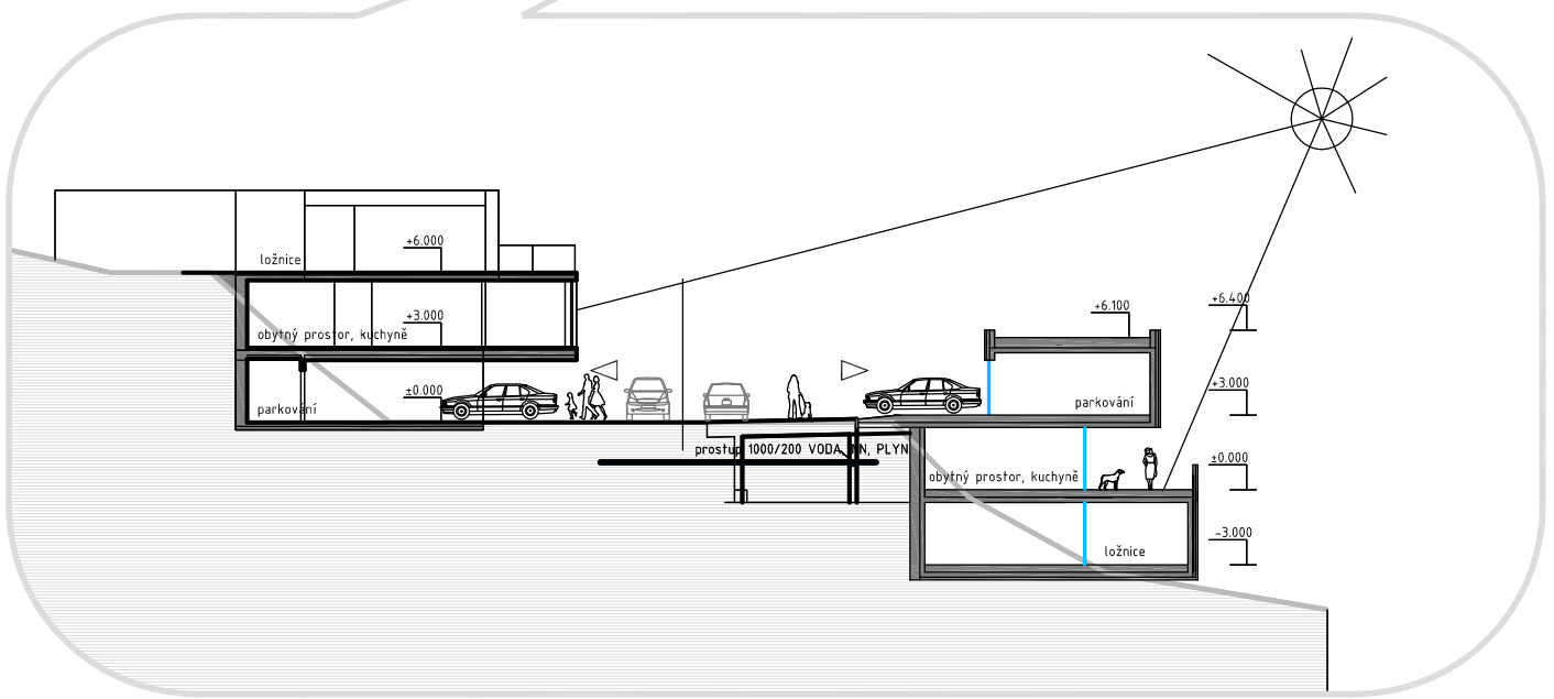
DETAIL SCHÉMATICKÉHO ŘEZU (HMOTOVÉ ŘEŠENÍ RODINNÝCH DOMŮ, VJEZDY, VÝŠKOVÉ ČLENĚNÍ DOMŮ) M 1:250
