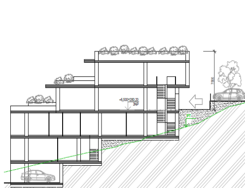
Řez a pohled - uvažovaná výstavba terasových bytových domů
