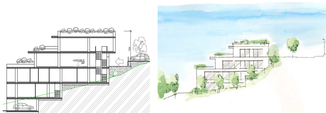
Řez a pohled - uvažovaná výstavba terasových bytových domů
